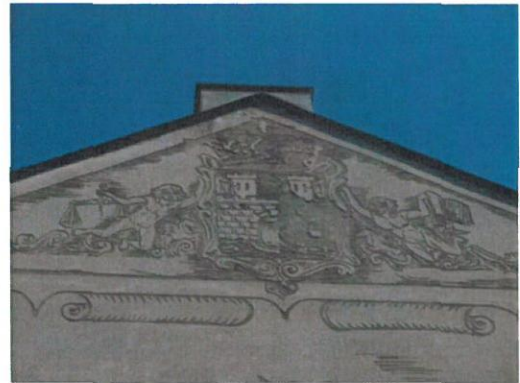
Sgraffito na elewacji budynku przy ul. Kraszewskiego 14 przed rozpoczęciem prac konserwatorskich.
